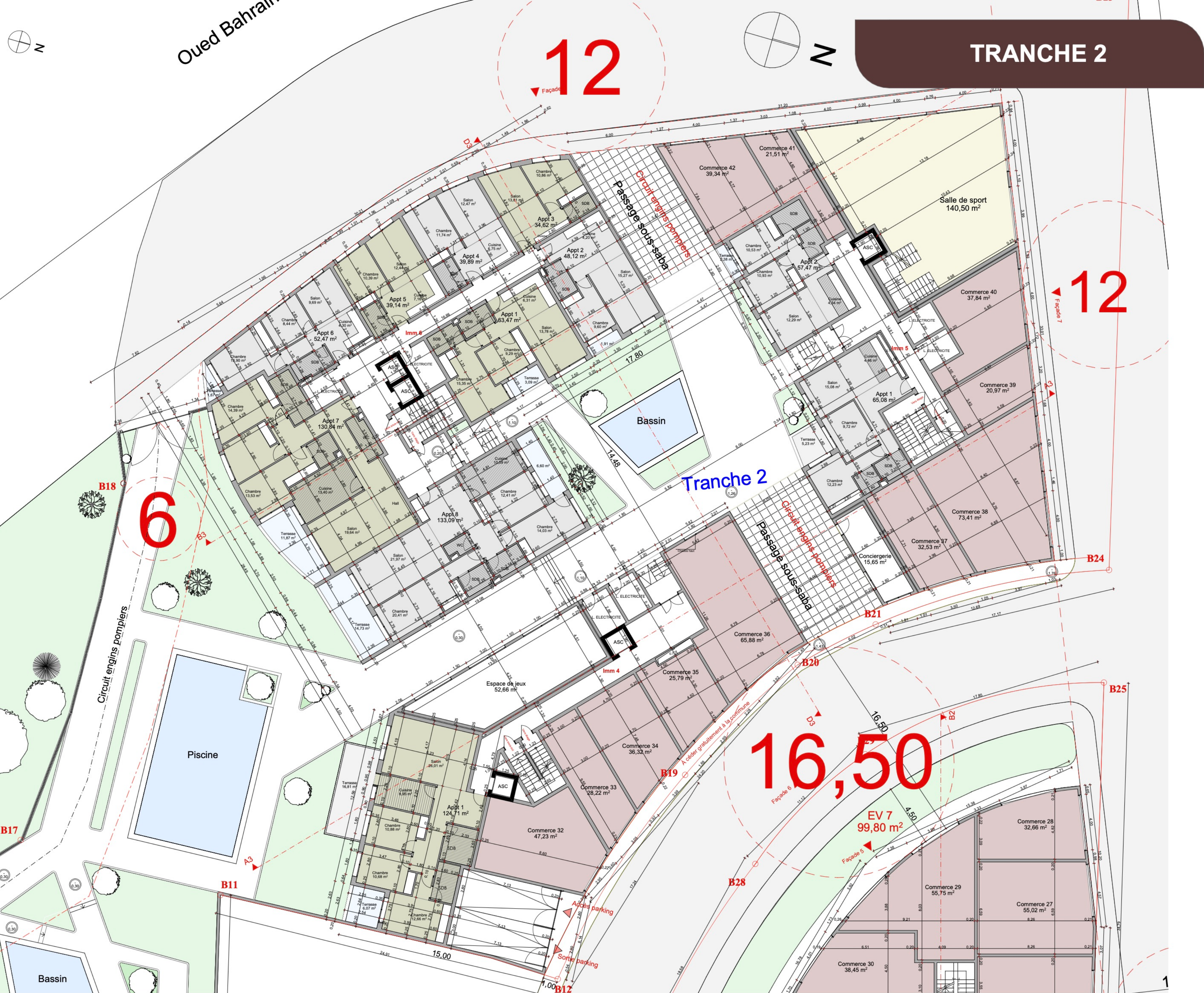
PLAN DU REZ-DE-CHAUSSÉE
